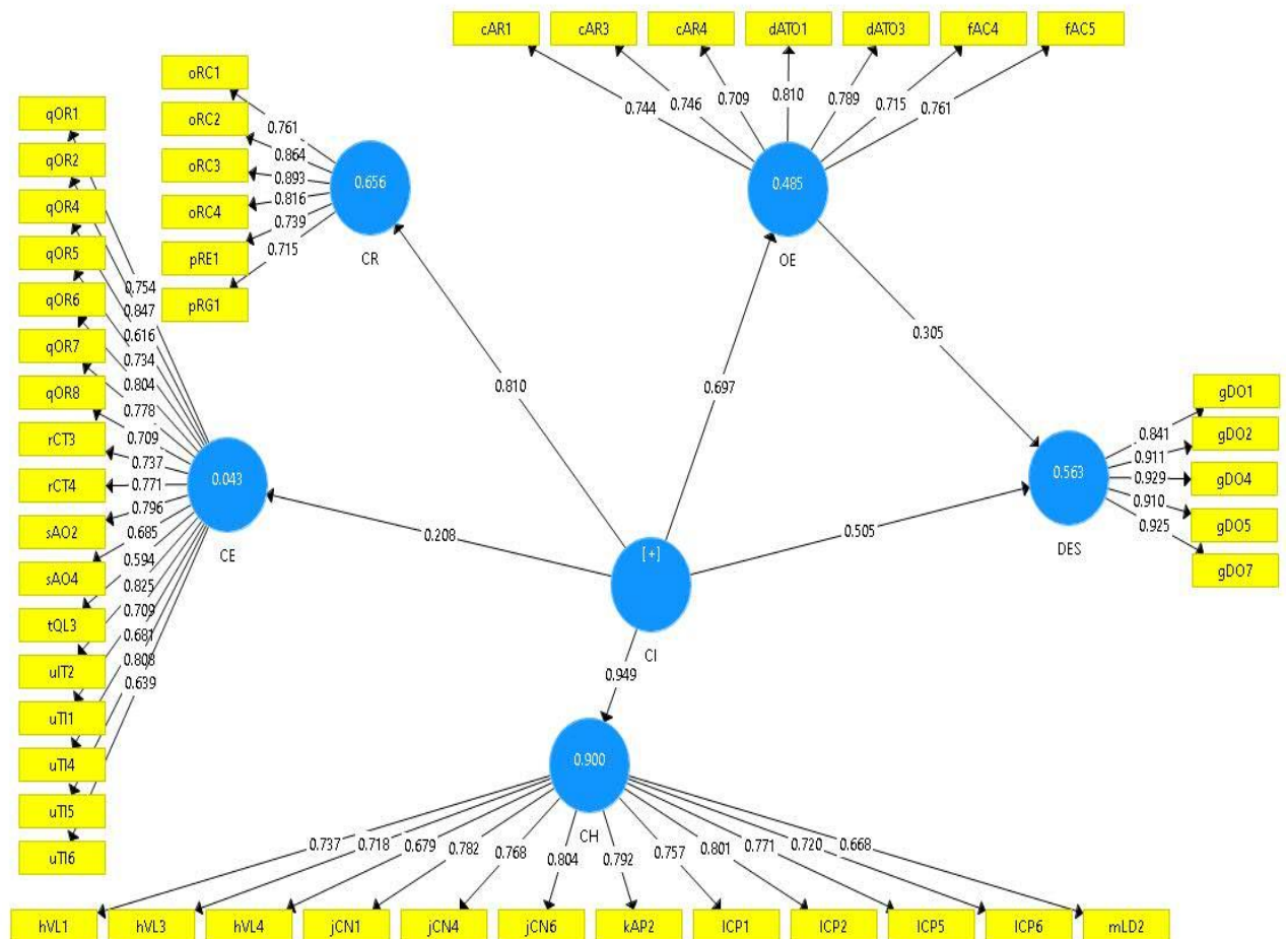
Figura 2: Modelo de mensuração e estrutural
