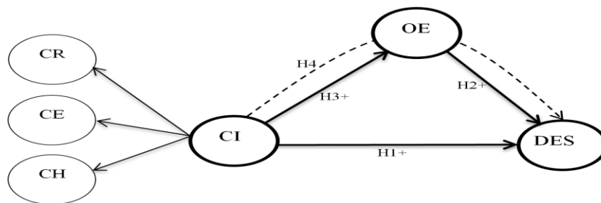
Figura 1 - Modelo teórico
